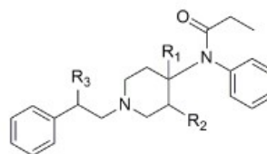
deriváty N -(1-fenethylpiperidin-4-yl)- N -fenylpropanamidu
